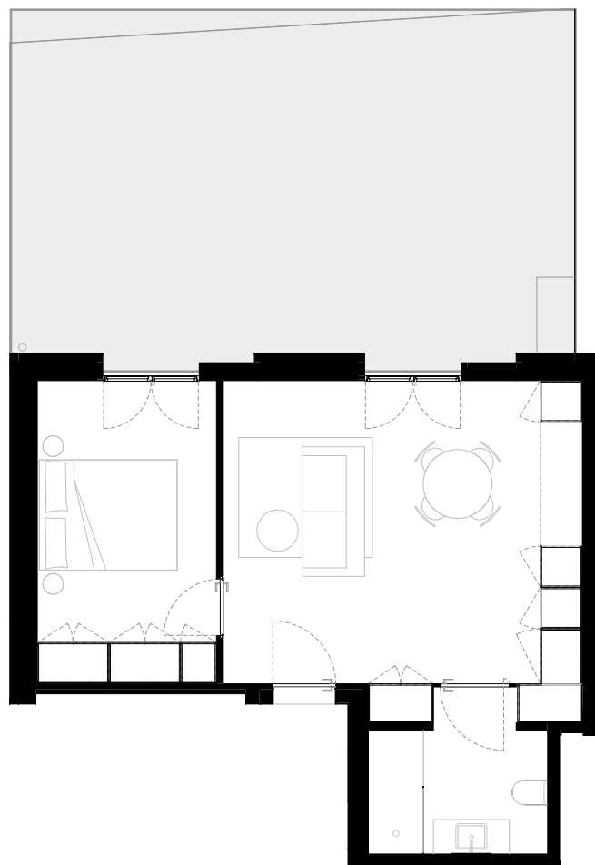
PISO 2 ESCALA 1:100
